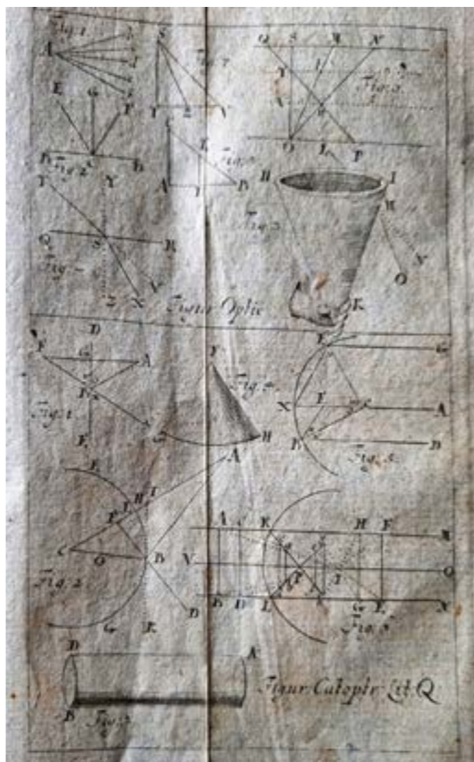
Geometriska figurer i detalj, från den gamla tyska matematikboken
